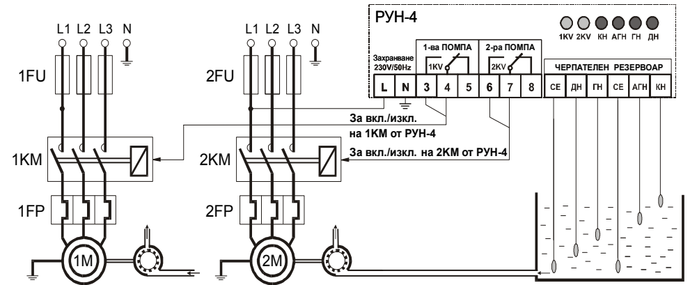
Фиг.1. Схема на присъединяване на РУН-4
